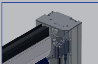
Oberer Sicherheitsendschalter
